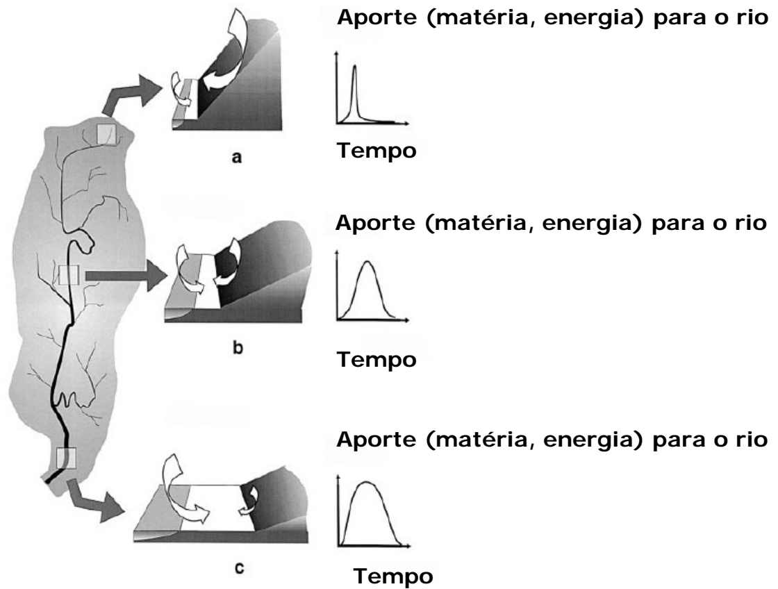
Figura 1. Entrada de informações no sistema (diagramas laterais) e principais setores de uma bacia hidrográfica, a) setor inicial ou erosivo; b) setor intermediário ou de transição; c) setor deposicional (modificado de Tabacchi et al. 1998).
