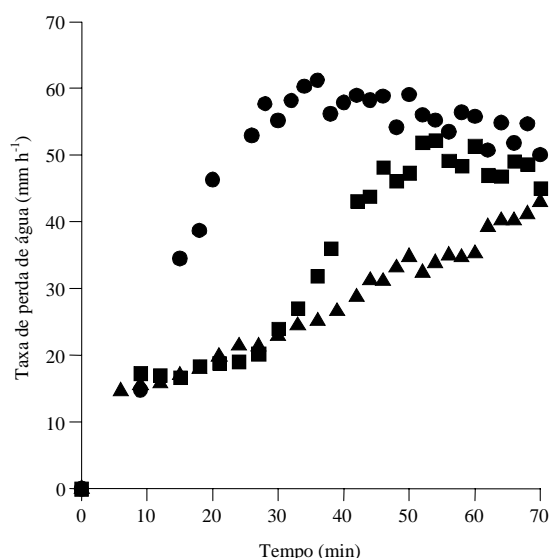
Figura 1. Taxa de perda de gua em entressulcos, em razo do tempo de aplicao da chuva simulada, nos diferentes tratamentos (●: preparo convencional com solo descoberto; ■: preparo convencional com palha incorporada; ▲: sem preparo). Media de seis repetioes.
