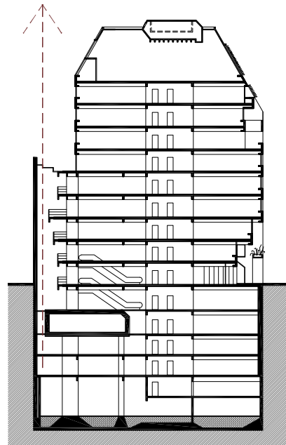
CORTE LONGITUDINAL
