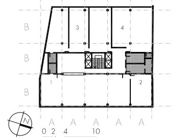
3º PISO
