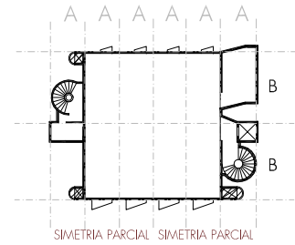
PLANTA BAIXA ESCRITÓRIOS
