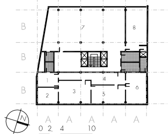
2º PISO
