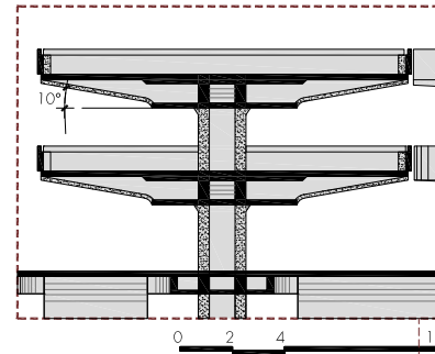
DETALHE BANDEJAS
