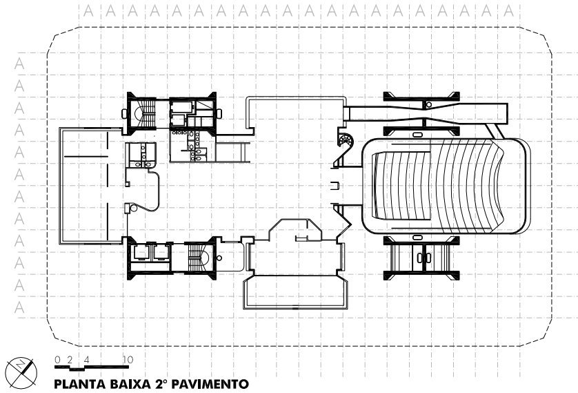
PLANTA BAIXA 2º PAVIMENTO
