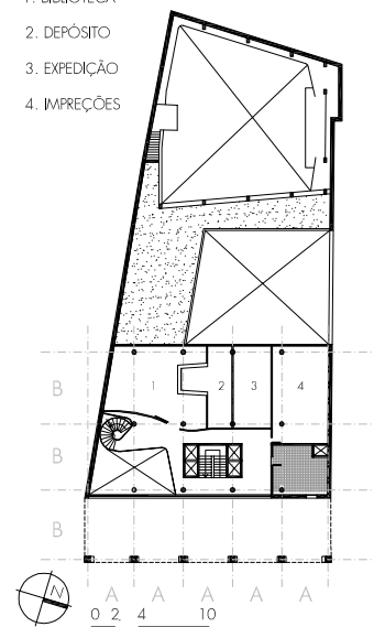
ENTREPISO
