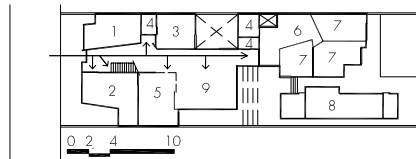
PLANTA BAIXA TÉRREO
