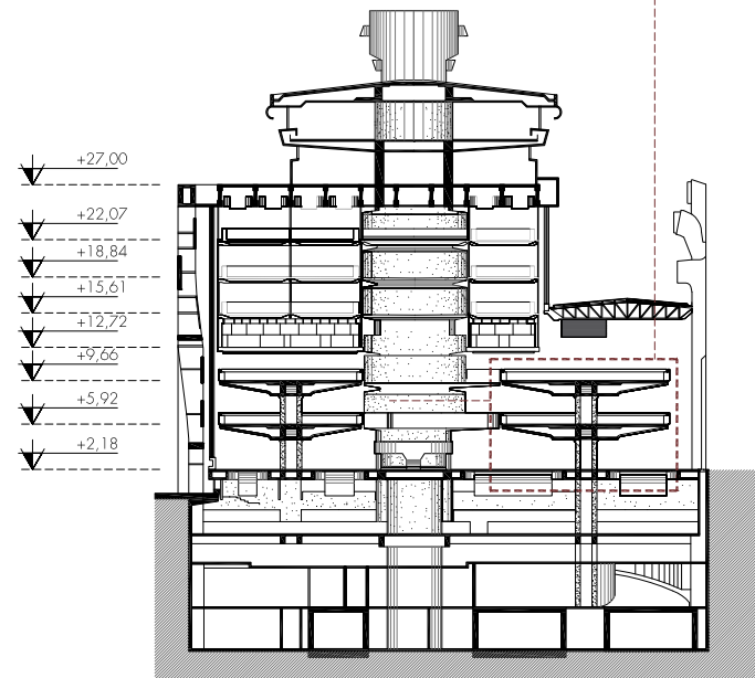
CORTE TRANSVERSAL
