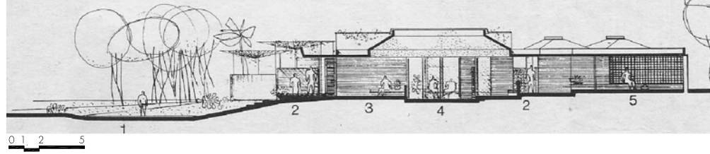
CORTE TRANSVERSAL AA - SETOR DE ESTAR E REFEITÓRIO
