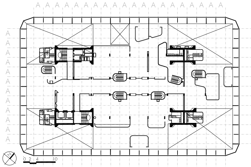
PLANTA BAIXA 3º PAVIMENTO
