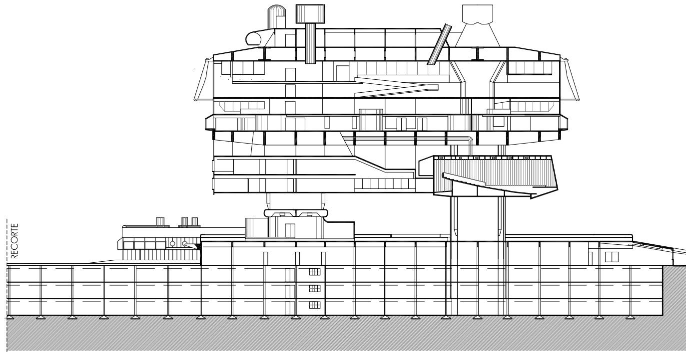
CORTE LONGITUDINAL
