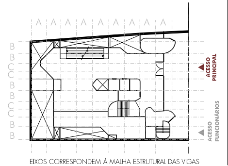
PLANTA BAIXA TÉRREO
