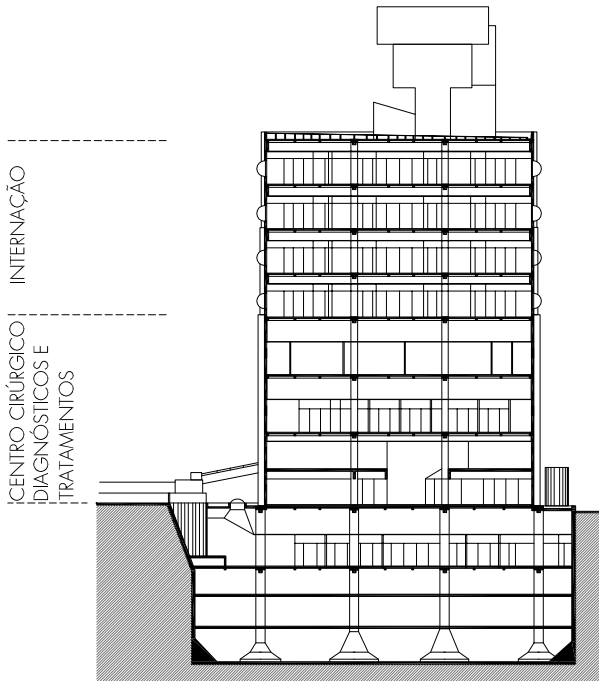
CORTE TRANSVERSAL
