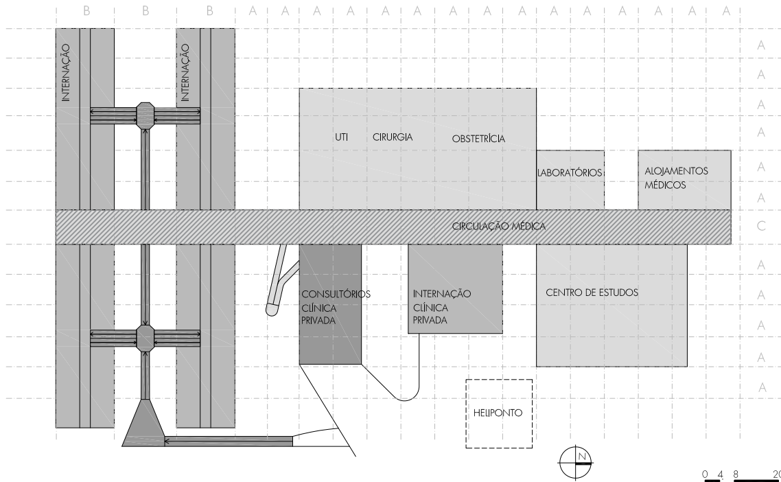
DIAGRAMA PLANTA BAIXA INTERNAÇÃO
