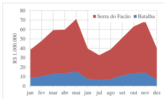
Figura 7 - Benefícios gerados pela geração de energia hidrelétrica para os 12 meses do ano com 10% de probabilidade de não excedência
