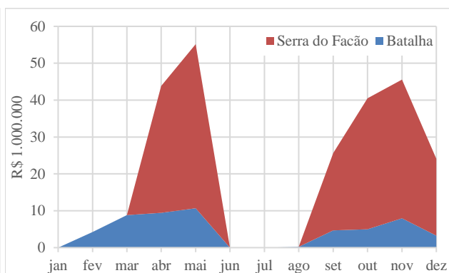
Figura 5 - Benefícios gerados pela geração de energia hidrelétrica para os 12 meses do ano com 90% de probabilidade de não excedência
