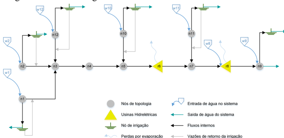
Figura 2 - Representação do sistema da bacia do São Marcos no modelo SDDP
