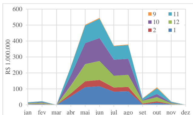
Figura 4 - Benefícios gerados pela agricultura irrigada nos nós de irrigação para os 12 meses do ano com 90% de probabilidade de não excedência
