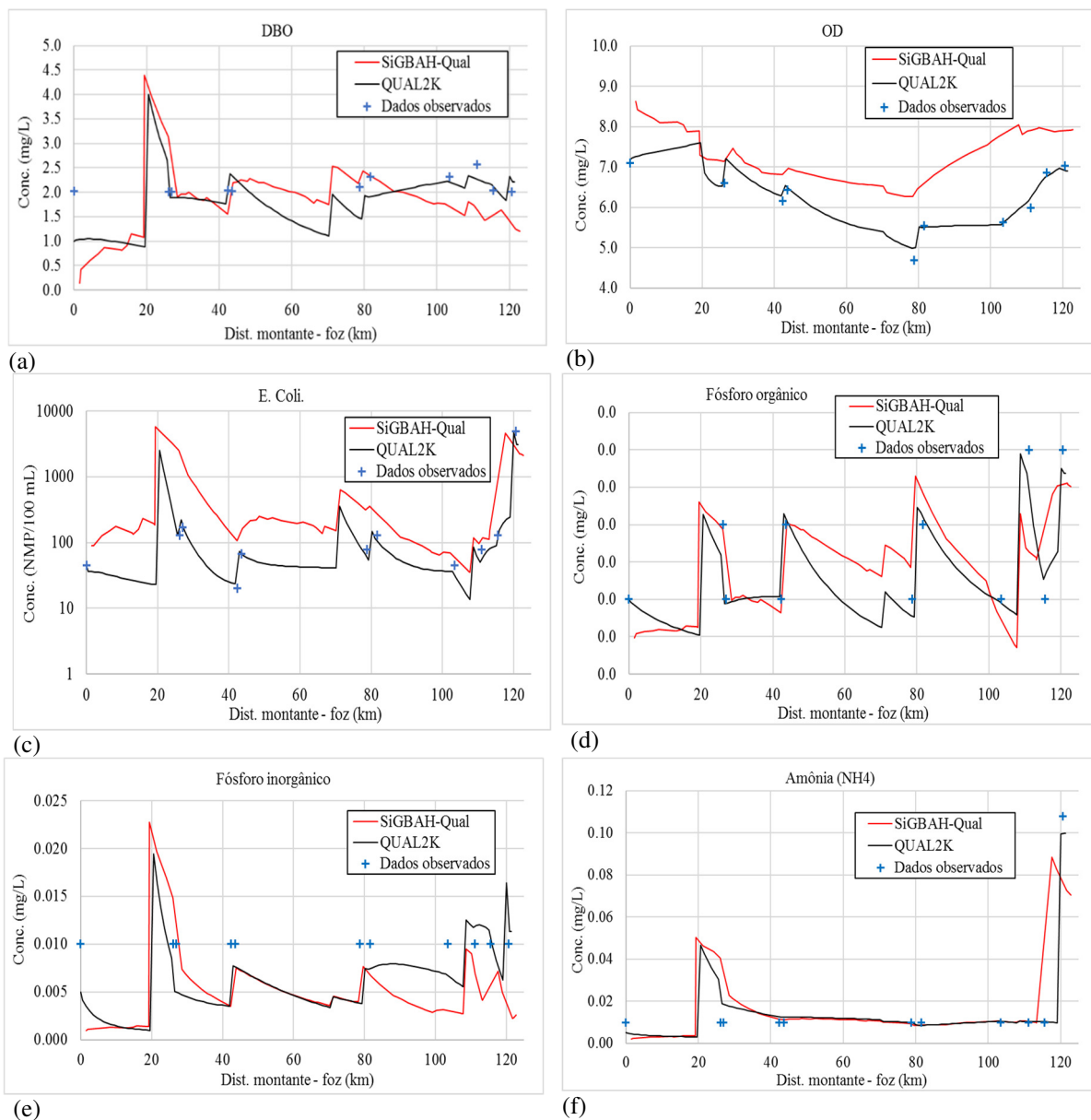
Figura 4 - Resultados da simulação do QUAL2-K e do SiGBAH-Qual ao longo do curso principal do rio Macaé para os seguintes parâmetros: a) DBO, b) oxigênio dissolvido, c) coliformes, d) fósforo orgânico, e) fósforo inorgânico e f) amônia.
