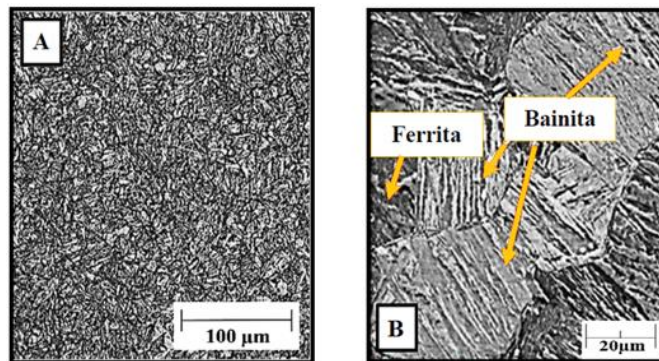
Figura 4: Micrografia em microscópio óptico em “A” (ampliação de 500x) e em MEV em “B” (ampliação de 10000x).
