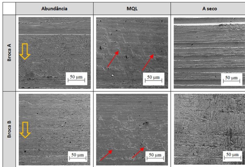
Figura 7: Superfície usinada na saída dos furos (ampliação 500x). As setas amarelas indicam o sentido de avanço da broca. As setas vermelhas apontam a zona de escorregamento com fluxo irregular de material deformado.
