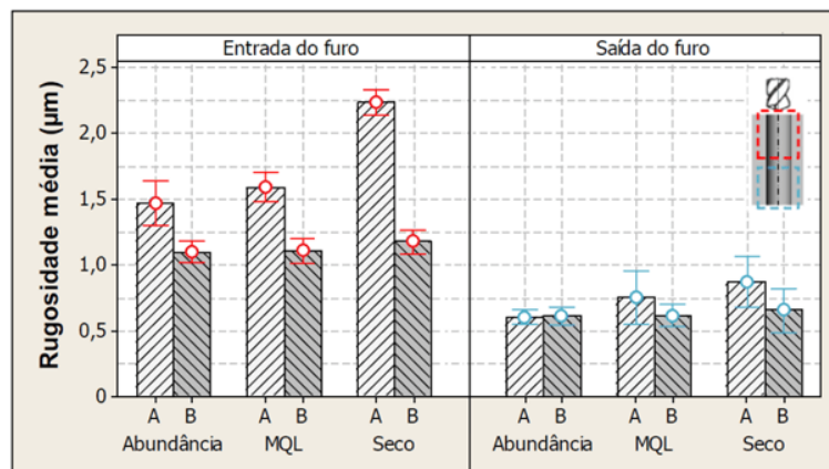
Figura 5: Valores de rugosidade para diferentes meios lubrificantes.
