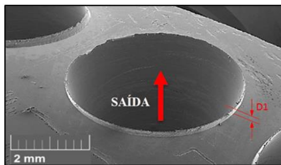
Figura 8: Topografia geral da rebarba gerada pelo processo de furação.
