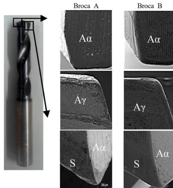
Figura 1: Imagens das brocas obtidas com MEV (ampliação 500x): face ( A\gamma ), flanco ( A\alpha ) e guia secundária (S).
