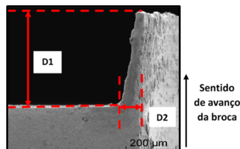
Figura 3: Esquema de orientação das medidas realizadas na rebarba gerada na saída dos furos: altura da rebarba (D1) e espessura da raiz (D2).
