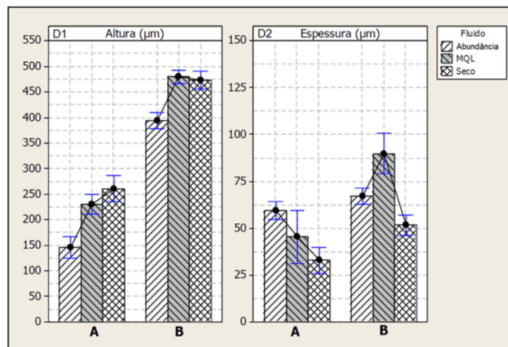
Figura 9: Valores médios da altura (D1) e espessura da raiz (D2) das rebarbas.
