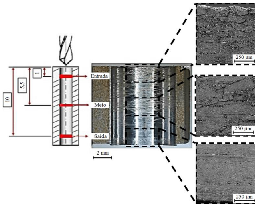
Figura 2: Representação das regiões de análise qualitativa das texturas dos furos.
