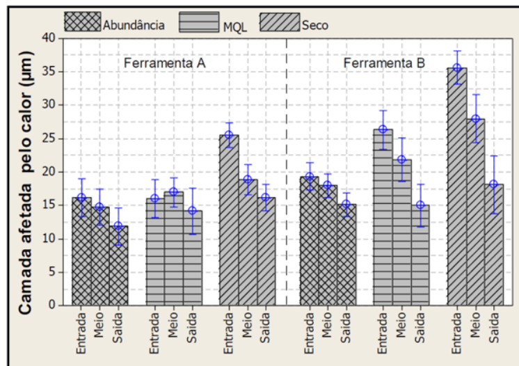
Figura 10: Valores médios da largura da camada afetada pelo calor (CAC).
