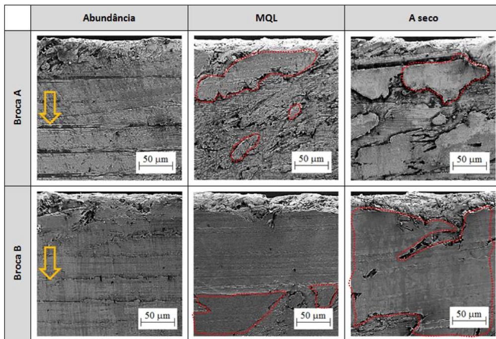
Figura 6: Superfície usinada na entrada dos furos (ampliação 500x). As setas amarelas indicam o sentido de avanço da broca. As linhas tracejadas em vermelho indicam o material aderido (caldeado) sobre a superfície do furo.
