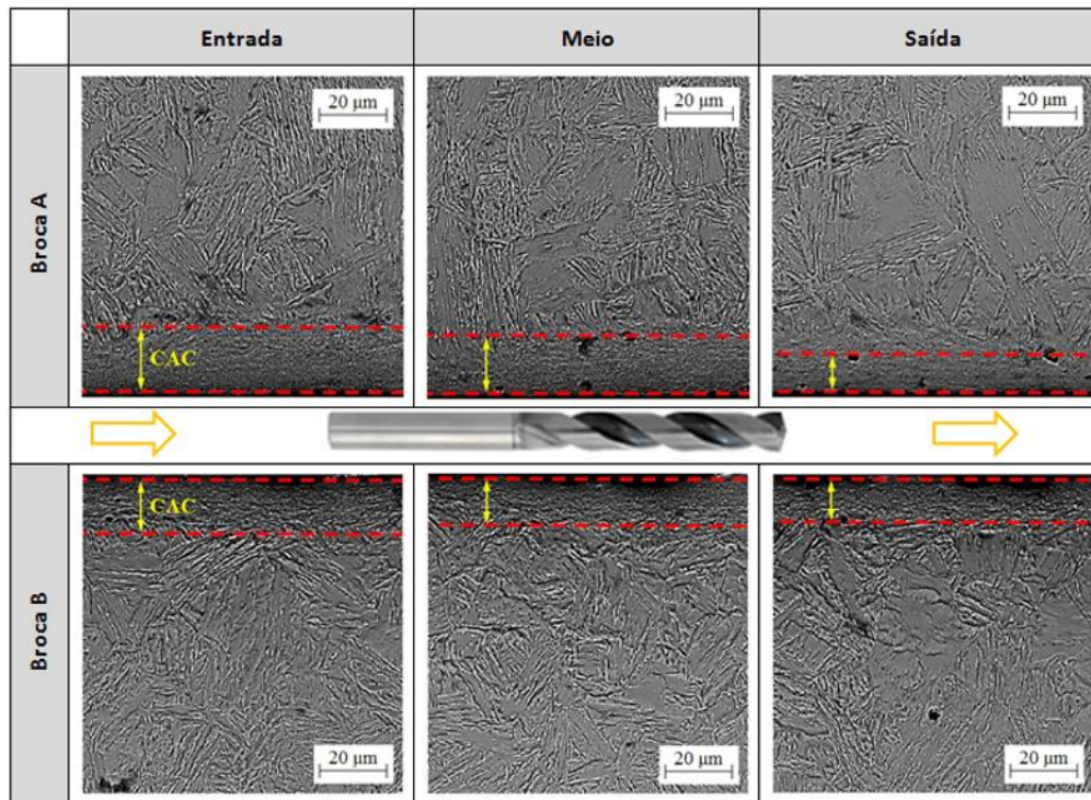
Figura 11: Representação da camada afetada pelo calor (CAC) para as brocas “A” e “B” na furação a seco.
