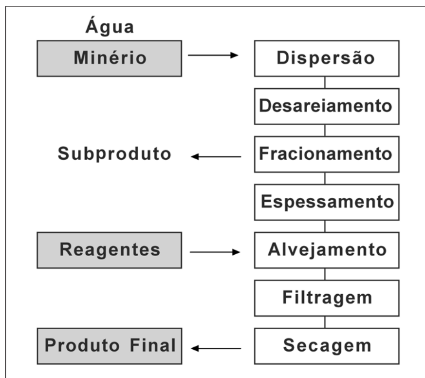
Figura 1 - Fluxograma generalizado do processamento do caulim.
