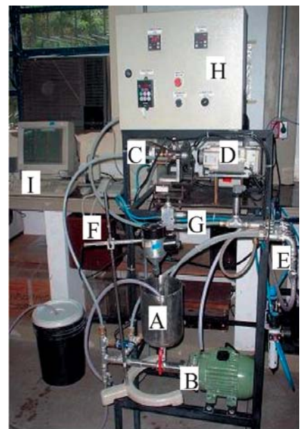
Figura 3 - Sistema Colorcell.
