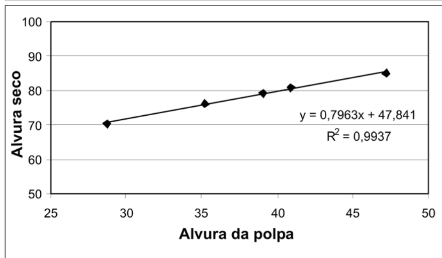
Figura 6 - Correlação entre os valores de alvura seca e úmida das amostras de caulim.
