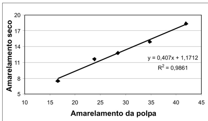
Figura 7 - Correlação entre os valores de amarelamento seco e úmido das amostras de caulim.
