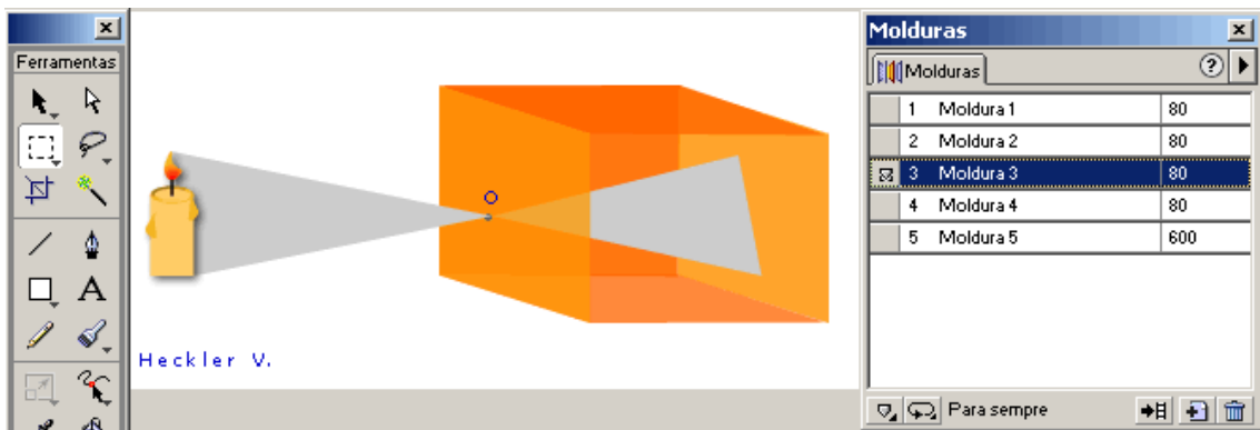
Figura 17 – Desenvolvimento da animação de formação da imagem na câmara escura, camada 3
