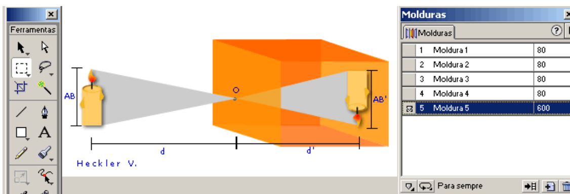
Figura 19 – Desenvolvimento da animação de formação da imagem na câmera escura, camada 5
