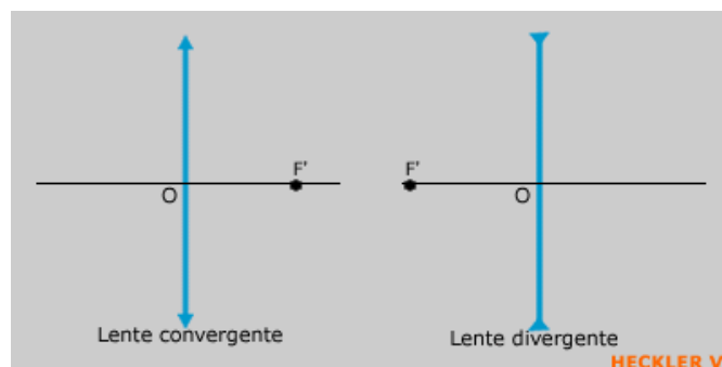
Simulação 8.2.1 - Simulação da convergência e da divergência dos raios emergentes de lentes delgadas.
