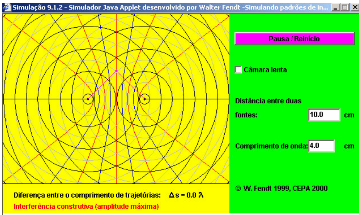
Simulação 9.1.2 - Simulando padrões de interferência produzidos por duas fontes vibrantes. Desenvolvido por Walter Fendt e traduzido pela CEPA -IFUSP - http://cepa.if.usp.br/walterfendt
