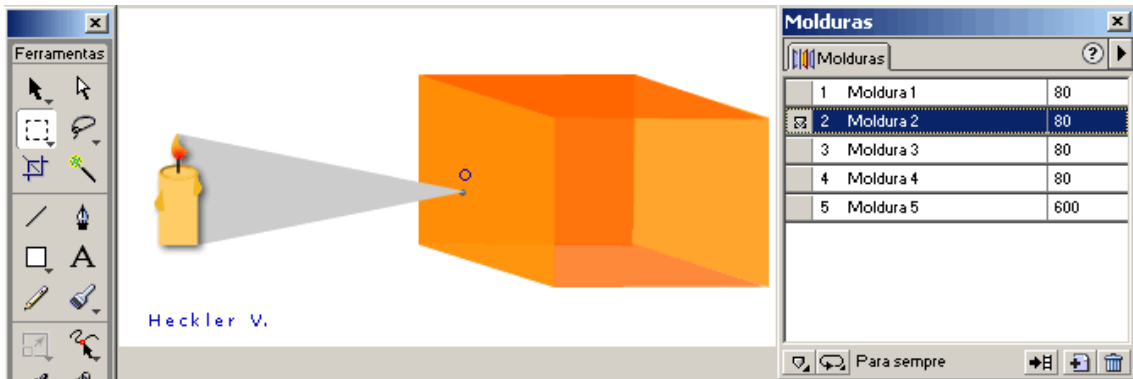
Figura 16 – Desenvolvimento da animação de formação da imagem na câmara escura, camada 2
