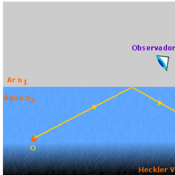
Figura 7.5.3 - O dióptro plano não produz imagens fora da região do ângulo limite.
