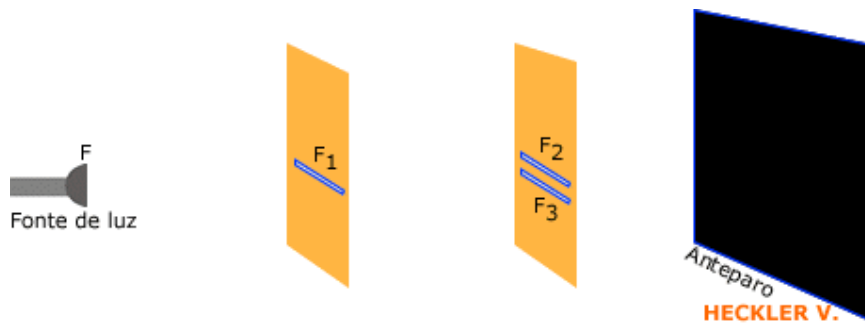
Simulação 9.2.1 - Simulando o experimento de Young, produzindo um padrão de interferência no anteparo.
