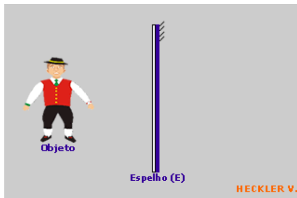
Simulação 5.3.1 - Simulando a formação de imagem de um objeto e um espelho plano.
