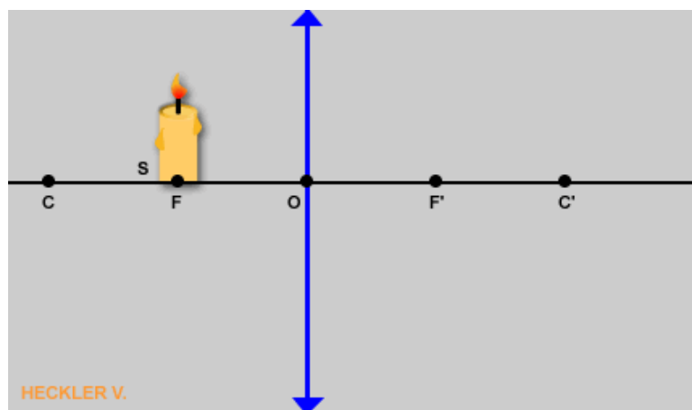
Simulação 8.2.7 - Simulando a possível formação da imagem para objeto localizado no foco principal objeto F.
