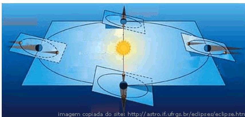
imagem copiada do site: http://astro.if.ufrgs.br/eclipses/eclipse.htm Figura 3.3.1 - Figura que mostra o plano da órbita da Lua em torno da Terra.
