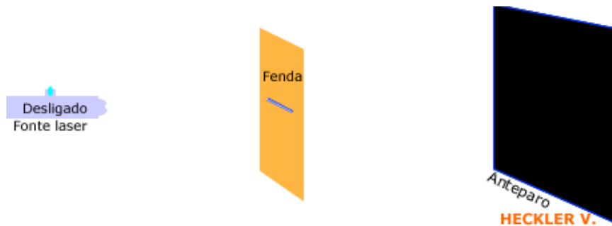
Simulação 10.1.2 - Difração: formação de regiões claras escuras pela luz do laser que passa por uma fenda estreita.
