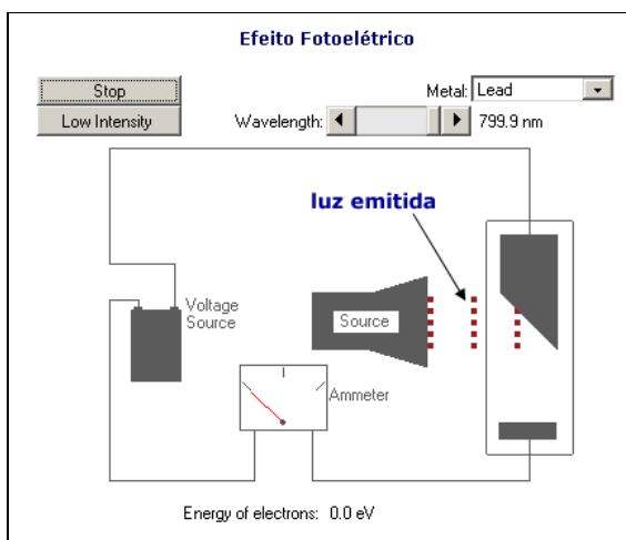
Figura 11 – Demonstração da não ejeção de elétrons
