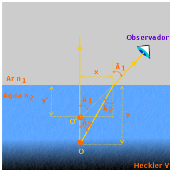
Figura 7.5.4 - Representação das relações angulares do dióptro plano.
