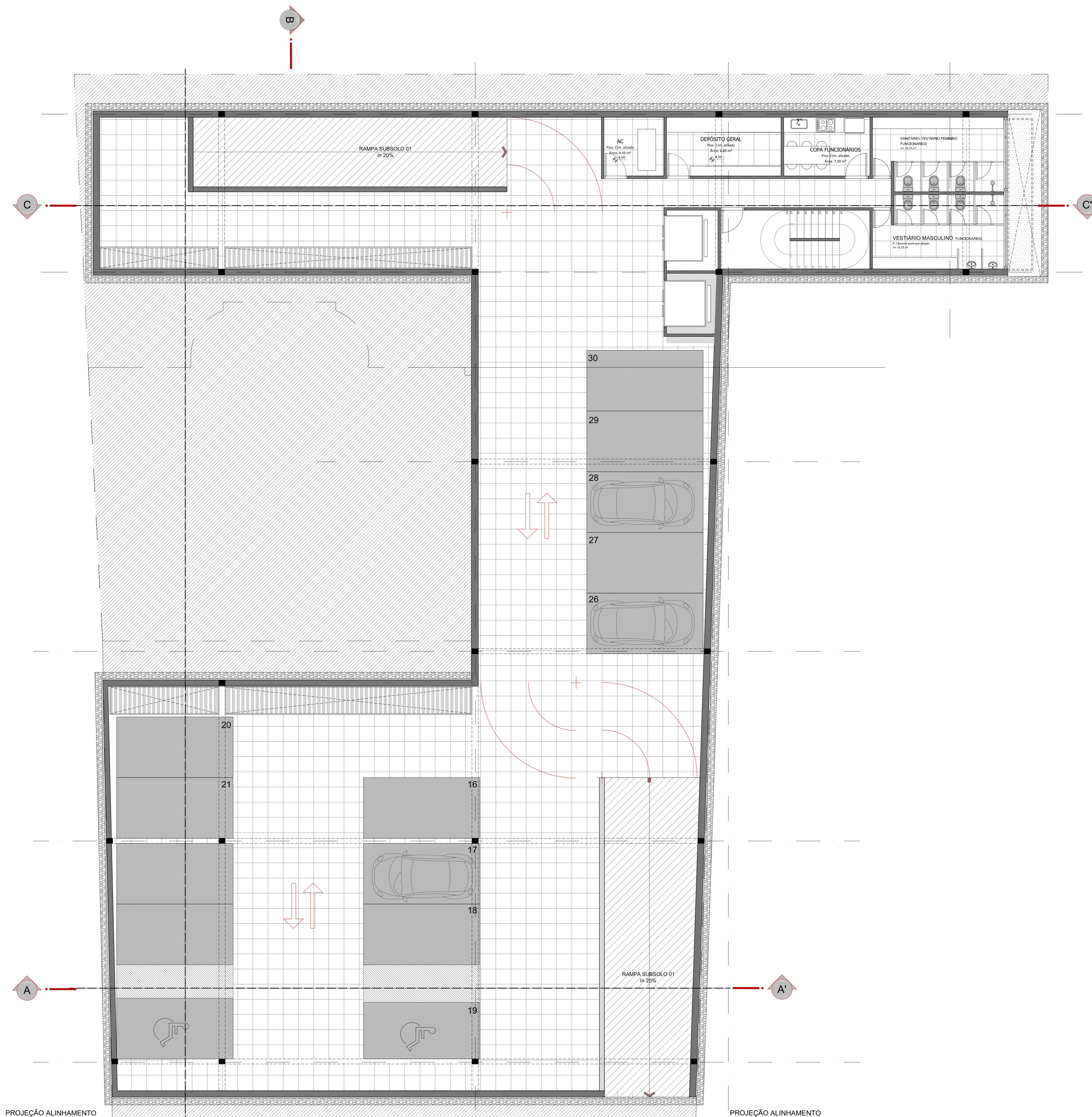
PLANTA BAIXA 2o SUBSOLO_esc 1/75
