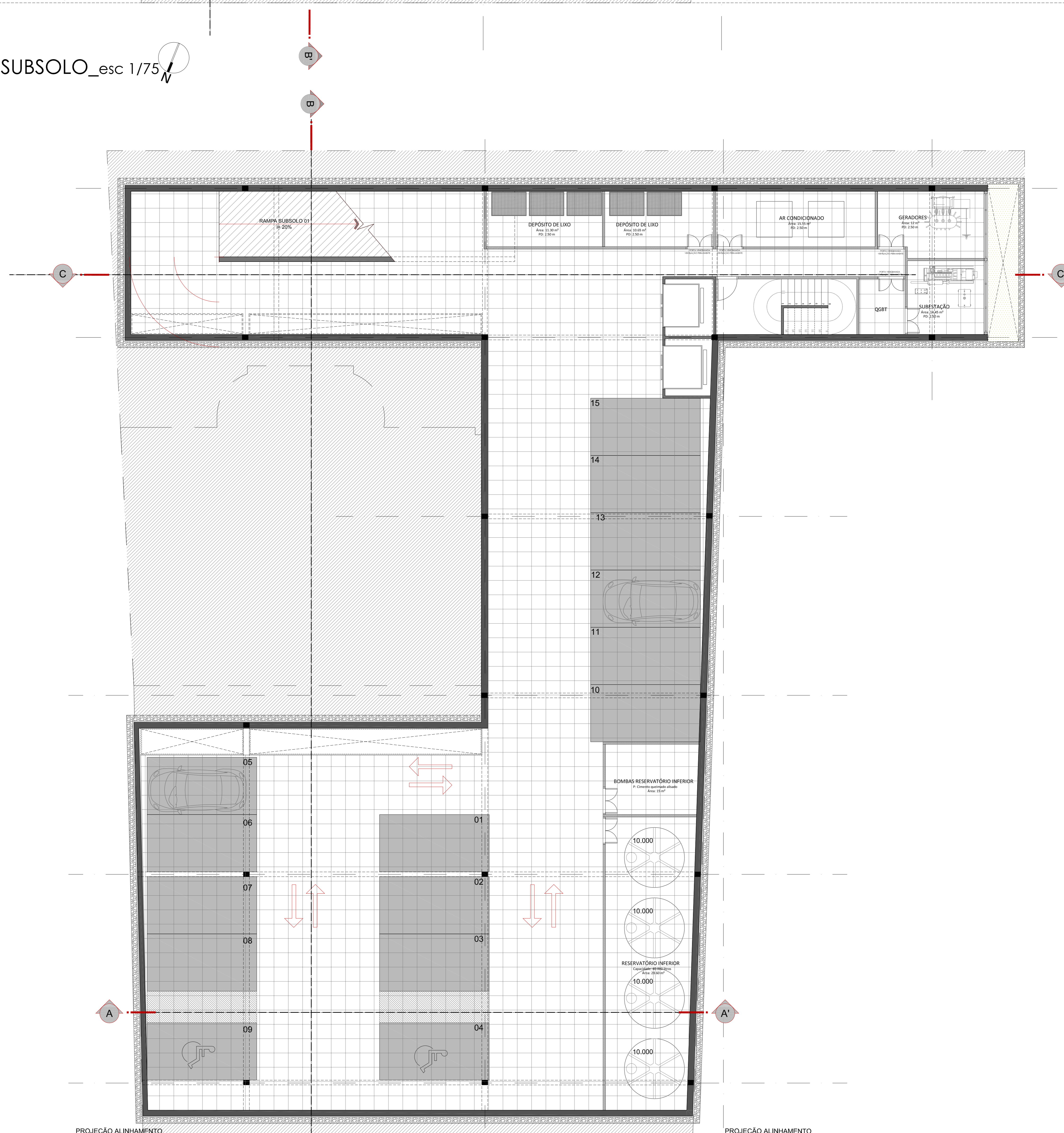
PLANTA BAIXA 1o SUBSOLO_esc 1/75
