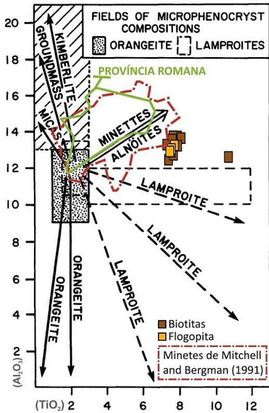
Figura 6.18 – Análises do Alfeu-I em gráfico de tendências de evolução composicional ( Al_2O_3 versus TiO_2 ) de micas. Os campos de dados dos minettes e da Província Romana foram traçados a partir de análises de Mitchell and Bergman (1991). Figura modificada de Mitchell (1995).
