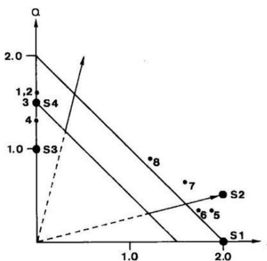
Figura 5.6 – Diagrama Q-J de Morimoto et al. (1988), onde ele exemplifica as composições de alguns piroxênios incomuns, numerados de 1 a 8 e com valores de “Q” menores que 1,62 e de Mn menor que 0,08 átomos por unidade de fórmula (cf. Tabela 3 em Morimoto 1988).
