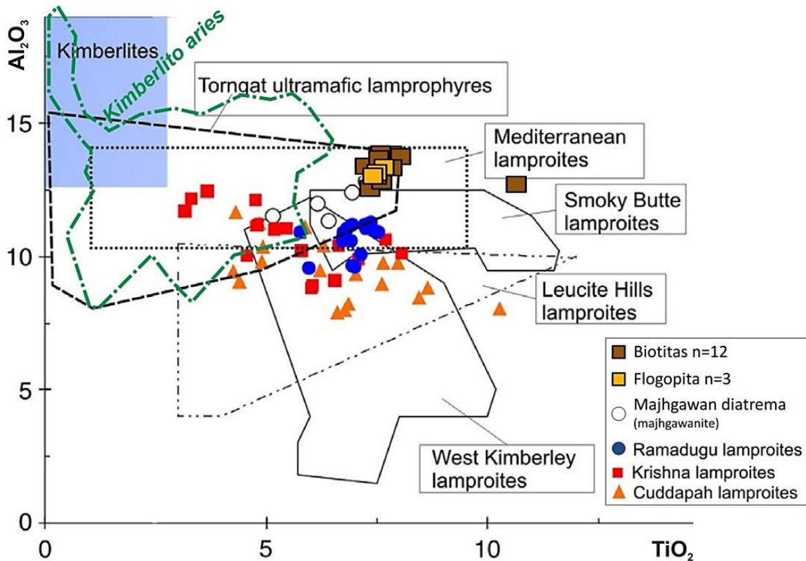
Figura 6.19 – Dados composicionais de Al_2O_3 x TiO_2 para as micas do Alfeu-I comparadas ao (s): dados para os lamproitos de Krishna, Majhgawan e Cuddapah, que são de Paul et al. (2007), Chalapathi Rao (2005) e Chalapathi Rao et al. (2010), respectivamente; campo das micas do lamprófiro ultramáfico de Torngat, de Tappe et al. (2004); kimberlito Aries, de Downes et al. (2006); campos de Leucite Hills, West Kimberley, Smoky Butte e lamproitos Mediterrâneos, obtidos de Chalapathi Rao et al. (2010) e de Fritschle et al. (2013), respectivamente. Figura modificada de Chalapathi Rao et al. (2014).
