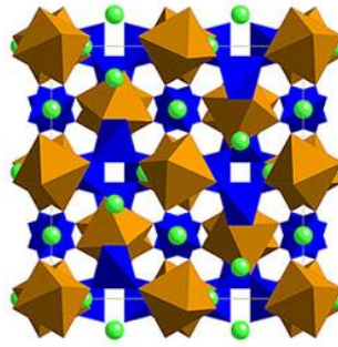
Figura 5.9 - Porção da estrutura tipo granada projetada ao longo do eixo z. Rede que exhibe a alternância entre sítios octaédricos (em marrom) e tetraédricos (em azul) e os cátions {X}, sítio dodecaédrico, representados em verde (obtida de GRAVINA, 2009).
