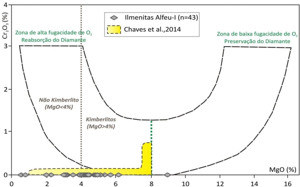
Figura 6.47 - Diagrama MgO x \text{Cr}_2\text{O}_3 de avaliação das condições de preservação e reabsorção de diamantes em ilmenitas (modificado de Haggerty, 1975 e Gurney e Moore, 1991).
