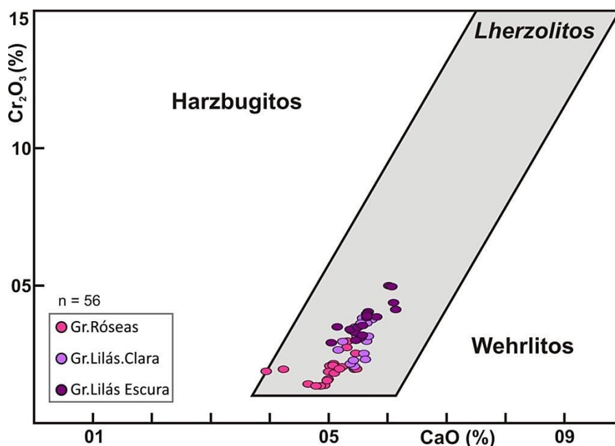
Figura 6.31 - Variação de CaO e \text{Cr}_2\text{O}_3 que classifica as granadas do Alfeu segundo os campos para peridotitos (lherzolitos, harzburgitos e wehrlitos). Granadas de lherzolitos ocorrem predominantemente na área sombreada dentro do polígono, figura modificada de SCHULZE (2003).
