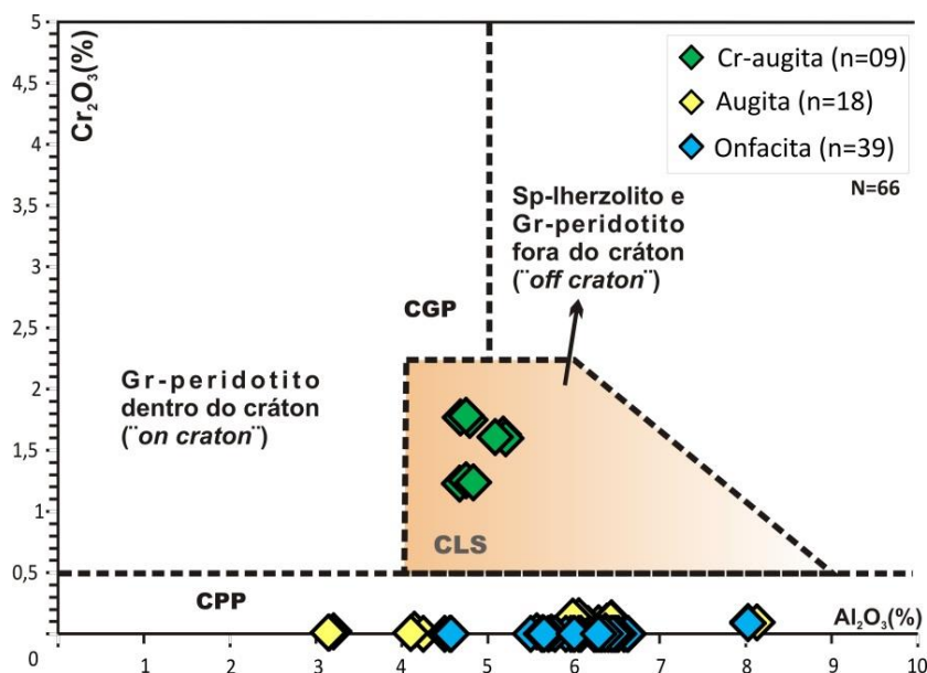
Figura 6.6 - Diagrama \text{Cr}_2\text{O}_3 vs. \text{Al}_2\text{O}_3 para todos os cpx analisados. CGP : é o campo de cpx derivados de manto granada peridotito "on-cráton". CLS : clinopiroxênios derivados de espinélio Iherzolito e de granada peridotitos "off-cráton". CPP : clinopiroxênios derivados de eclogitos, piroxenitos e megacristais. (Gr=granada, Sp=espinélio). Modificada de Ramsay e Tompkins (1994) e Silveira (2006).
