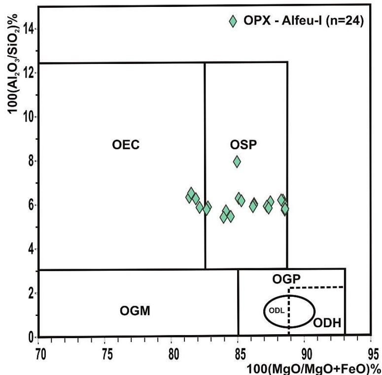
Figura 6.14 – Diagrama 100(Al_2O_3/SiO_2)\% v.s. 100(MgO/MgO+FeO)\% que discrimina campos de diferentes composições de rocha fonte para química de ortopiroxênios: ODH – opx de harzburgitos diamantíferos; ODL – opx de lherzolitos diamantíferos; OEC – opx de xenólitos eclogíticos/piroxeníticos; OGP – opx de granada peridotitos de localidades cratônicas; OGM – opx de granada peridotitos e megacristais de localidades cratônicas; OSP – opx de espinélio lherzolitos. Modificada de Ramsay e Tompkins (1994).
