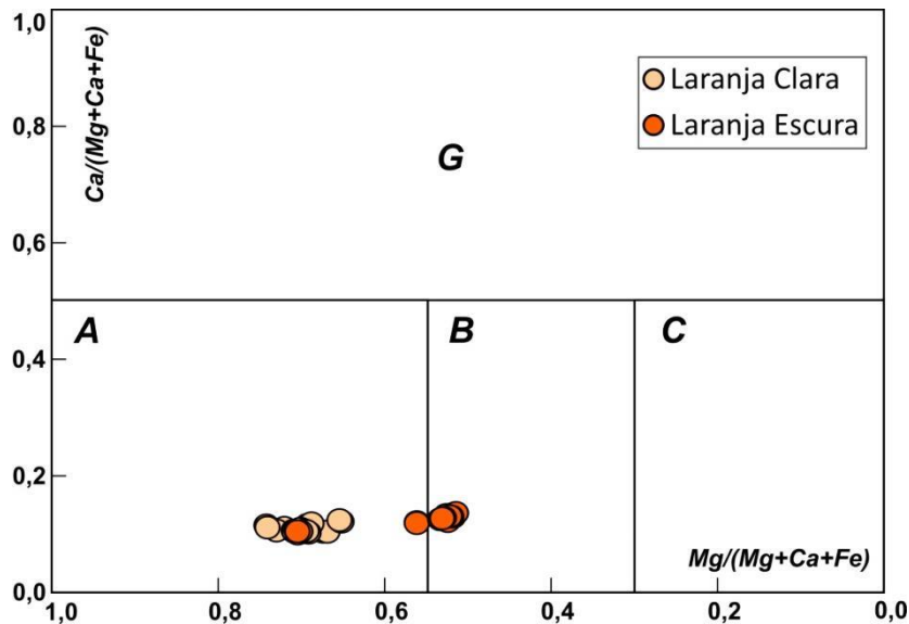
Figura 6.29 – Razões Mg/(Mg+Ca+Fe) \times Ca/(Ca+Mg+Fe) , em a.p.f.u, utilizada para subdividir as composições de granada eclogítica. Campo G (granadas de "Grospiditos") e aquelas com menores teores de cálcio (<50), subdivididas entre os grupos A, B e C. Modificada de SCHULZE (2003).
