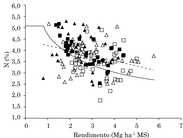
Figura 4. Curva de diluição de nitrogênio (-) e relação entre teor de N e rendimento da cultura de soja fertilizada pela adubação sistêmica em Sistemas Integrados de Produção Agropecuária (—) ( \hat{y} = 4,6 - 0,288 x ; p < 0,0001 ; R^2 = 0,1735 ; DPR = 0,65 ; n = 190 ). Tratamentos: □ Contínuo moderada; ■ Rotativo moderada; △ Contínuo baixa; e ▲ Rotativo baixa.
