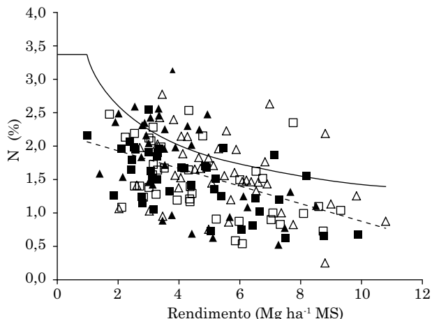
Figura 3. Curva de diluição de nitrogênio (-) e relação entre teor de N e rendimento da cultura de milho fertilizada pela adubação sistêmica em Sistemas Integrados de Produção Agropecuária (—) ( \hat{y} = 2,21 - 0,132 x ; p < 0,0001 ; R^2 = 0,2280 ; DPR = 0,50 ; n = 159 ). Tratamentos: □ Contínuo moderada; ■ Rotativo moderada; △ Contínuo baixa; e ▲ Rotativo baixa.
