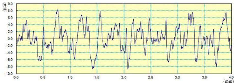
Figura 10: Perfil de rugosidade da barra 13a, típico para as amostras do grupo IG.
