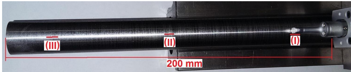
Figura 4: Posições de leitura da rugosidade para cada amostra.
