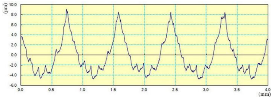
Figura 13: Perfil de rugosidade da barra 15a medida próximo ao centro da barra, região II.
