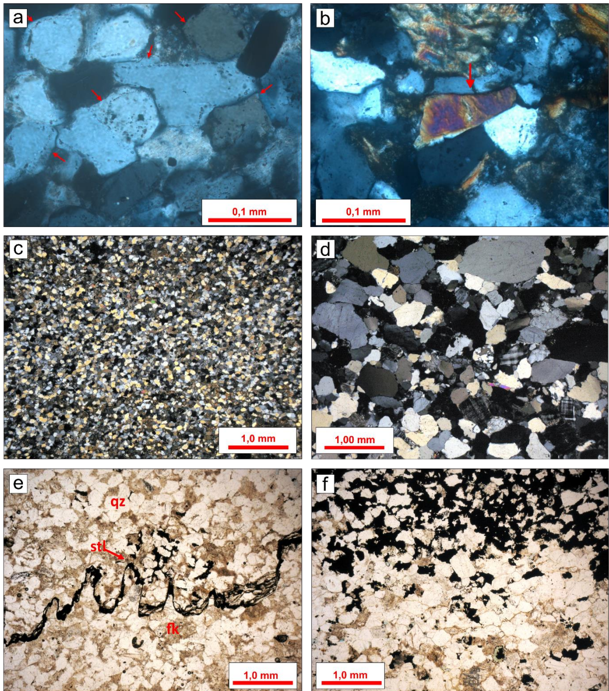
Figura 6. Fotomicrografias das lâminas petrográficas dos testemunhos de sondagem. a Lâmina ARASC9.1 apresenta intercrescimento de quartzo, situada antes da camada de carvão (luz polarizada, objetiva de 50x); b Lâmina ARASC9.2 destaca a presença de turmalina dendrítica, situada após a camada de carvão (luz polarizada, objetiva de 50x); c Lâmina ARASC10.3 apresenta porosidade nula e granulometria dos minerais fina, situada antes da camada de carvão (luz polarizada, objetiva de 25x); d Lâmina ARASC10.4 também apresenta porosidade nula, mas granulometria grossa, situada após a camada de carvão (luz polarizada, objetiva de 25x); e Lâmina ARASC14_5.1 mostra estilólitos e porosidade nula, camada associada ao carvão ausente no perfil (luz natural, objetiva de 25x); f Lâmina ARASC14_5.2 mostra a presença de opacos em aprox. 50% da lâmina (minerais pretos), camada associada ao carvão ausente no perfil (luz natural, objetiva de 25x).
