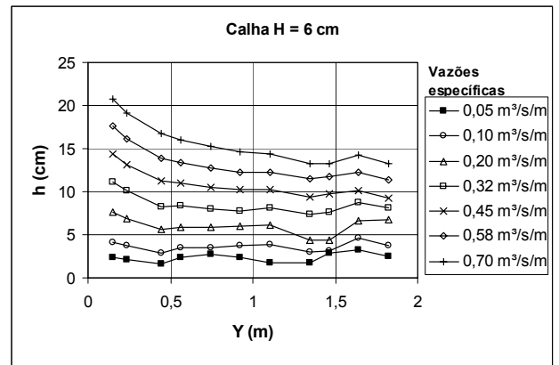
Figura 5 – Profundidade do escoamento ao longo da calha para as três estruturas em degraus, para os diferentes valores de vazões específicas ensaiados em cada estrutura.
