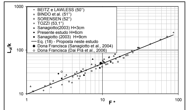
Figura 4 – Comparação da posição do início da aeração do escoamento entre os resultados obtidos no presente estudo, com os dados de outros pesquisadores (de acordo com Chanson 1994a, a equação (18), proposta neste estudo e um resultado obtido no vertedouro em degraus da UHE de Dona Francisca e de Val de Serra).
