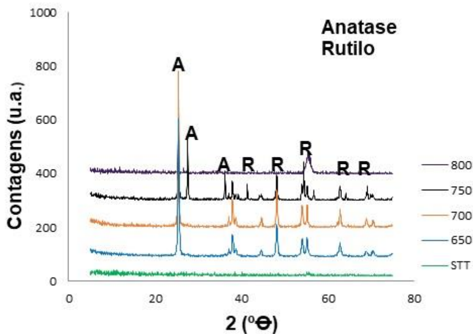
Figura 3. Difratograma das fibras de \text{TiO}_2 tratadas termicamente a 650^\circ\text{C} , 700^\circ\text{C} , 750^\circ\text{C} e 800^\circ\text{C} .
