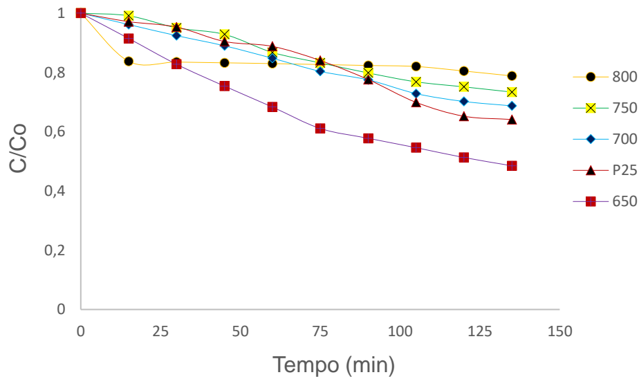
Figura 5. Concentração relativa do corante alaranjado de metila na presença de 50 mg de catalisador (fibras de TiO 2 ).
