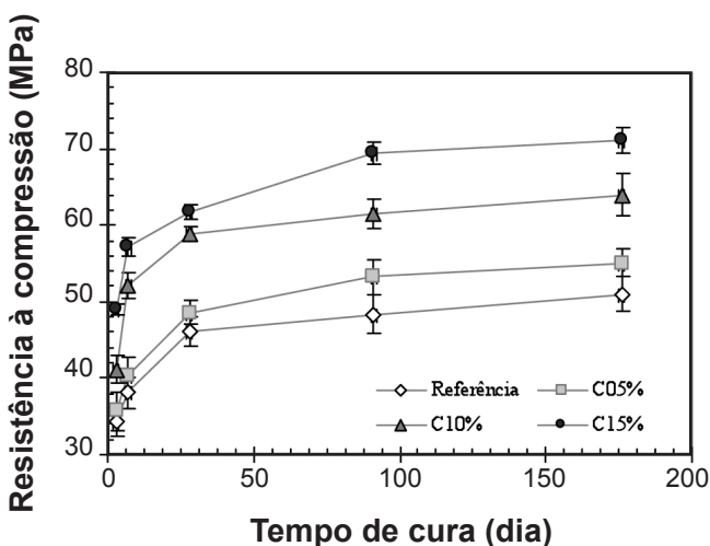
Figura 5: Resistência à compressão dos concretos com argila calcinada a 650 °C.
