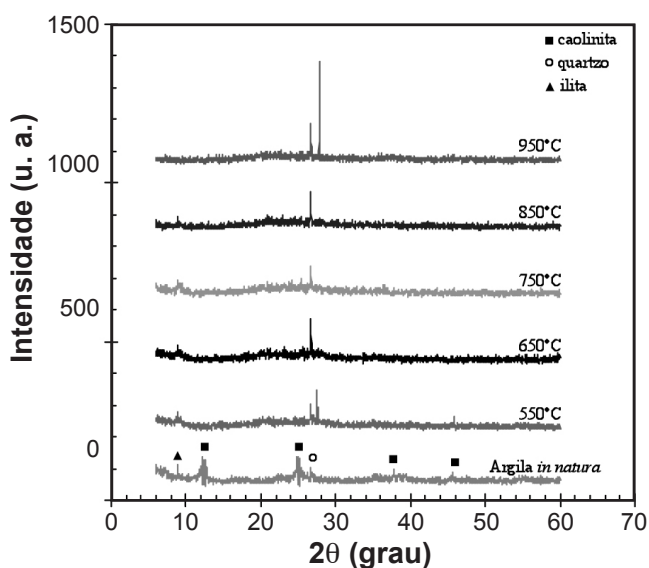
Figura 1: Difratoogramas de raios X das argilas in natura e calcinadas.
