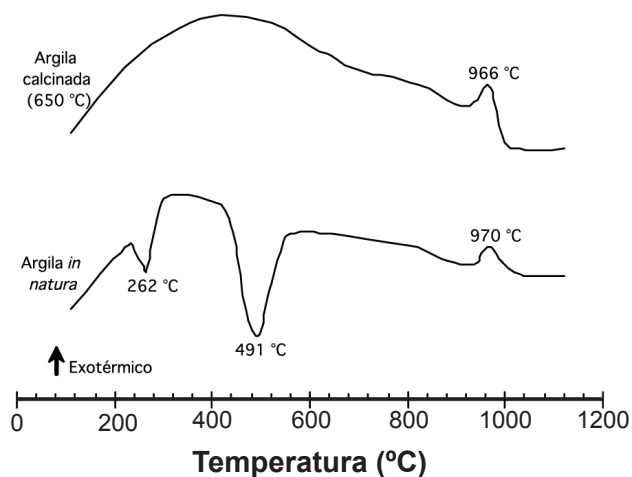
Figura 3: Curvas de análise térmica diferencial das argilas in natura e calcinada a 650 °C. Condições experimentais: taxa de aquecimento - 10 °C/min; sensibilidade - 100 \mu\text{m} ; termopar - Pt-Rh; inerte - \text{Al}_2\text{O}_3 . [Figure 3: DTA curves of in natura clay and calcined clay at 650 °C. Experimental conditions: heating rate - 10 °C/min; sensibility - 100 \mu\text{m} ; thermocouple - Pt-Rh; inert - \text{Al}_2\text{O}_3 .]
