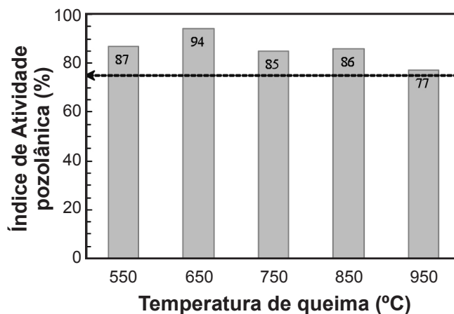
Figura 4: Índices de atividade pozolânica das argilas calcinadas. A linha tracejada representa o valor mínimo que caracteriza um material com pozolânica de acordo com a NBR 12653 [18]. [Figure 4: Pozzolanic activity indices of calcined clays. The dotted line represents the minimum value that characterizes a material as pozzolanic according to NBR 12653 [18].]
