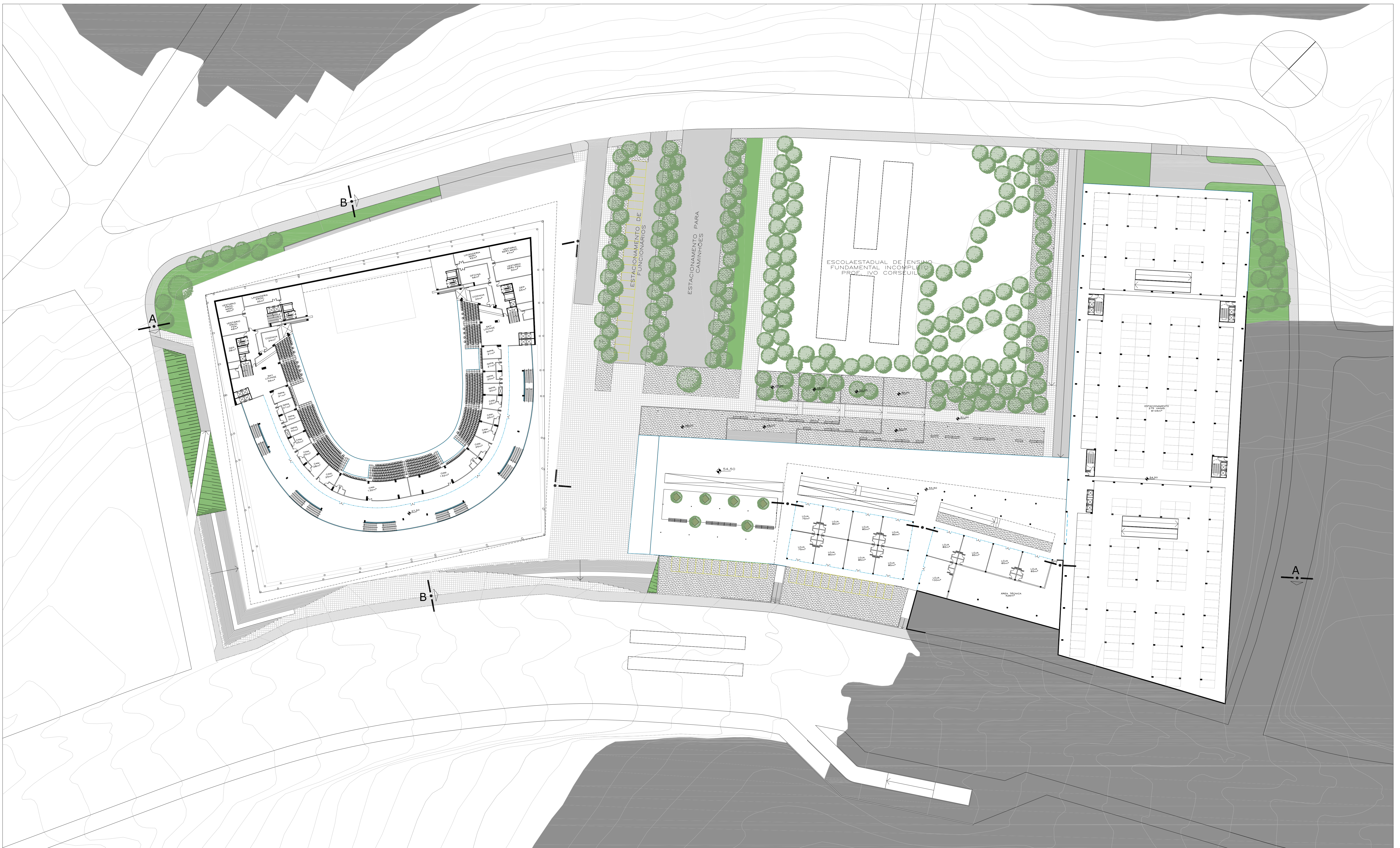
ARENA - NÍVEL 3 ESTACIONAMENTO - NÍVEL 4 LOJAS ESC. 1:500
