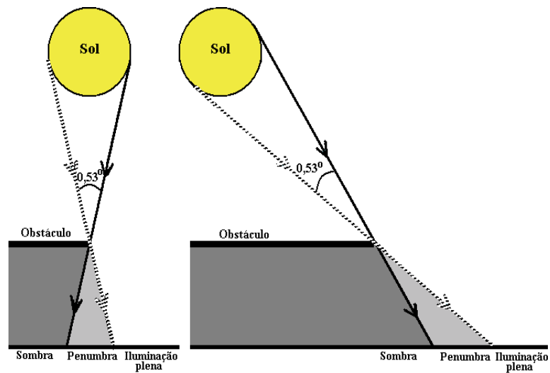
Fig. 8 - A luz solar que se origina em regiões diferentes do disco solar produz sombras com bordas não definidas, contornadas por uma região de penumbra.
