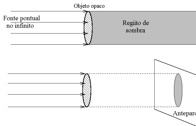
Fig. 4 - Para uma fonte pontual no infinito: região de sombra e a sombra sobre um anteparo. O tamanho da sombra não varia com a distância entre o objeto opaco e o anteparo.
