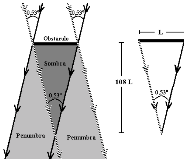
Fig. 9 - Representação esquemática da região de sombra produzida por um obstáculo que impede a passagem dos raios luminosos solares.
