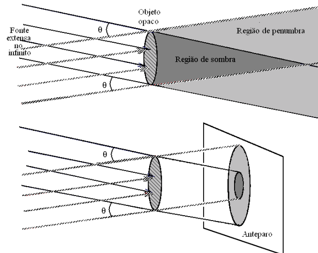
Fig. 7 - Sombra produzida por uma fonte extensa infinitamente distante. Linhas contínuas representam raios provindos do bordo superior da fonte; linhas pontilhadas, os raios provindos do bordo inferior.
