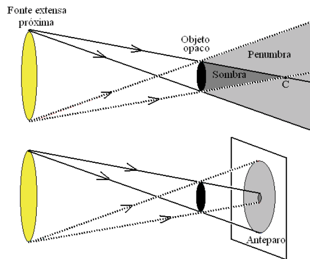
Fig. 5 - Sombra produzida por uma fonte extensa próxima e maior do que o objeto opaco que intercepta seus raios luminosos. A sombra em um anteparo é sempre menor do que o obstáculo, pois a seção transversal da região de sombra diminui conforme aumenta a distância ao obstáculo, ao passo que a seção da região de penumbra aumenta.
