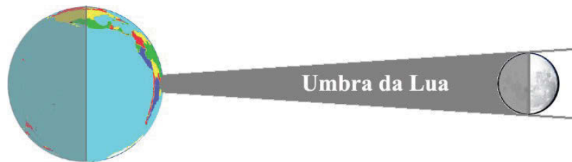
Fig. 11 - O vértice do cone de sombra ou umbra da Lua se encontra sempre próximo à superfície da Terra durante um eclipse solar total, determinando que o diâmetro da sombra da Lua na Terra seja muito menor do que o diâmetro lunar.
