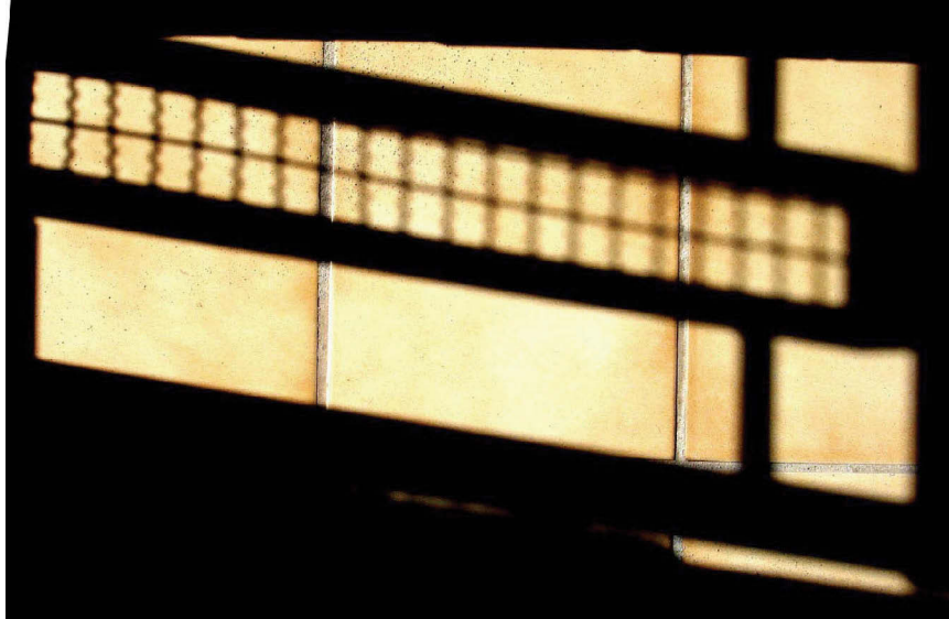
Fig. 10 - Grade de arame intercepta a luz solar produzindo sombra e penumbra.
