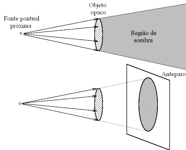
Fig. 3 - Sombra produzida por uma fonte pontual próxima: a região de sombra e a sua seção transversal, como aparece ao incidir a luz da fonte em um anteparo. A sombra é tanto maior quanto mais distante do anteparo estiver o objeto opaco, e quanto mais próxima deste se encontrar a fonte.
