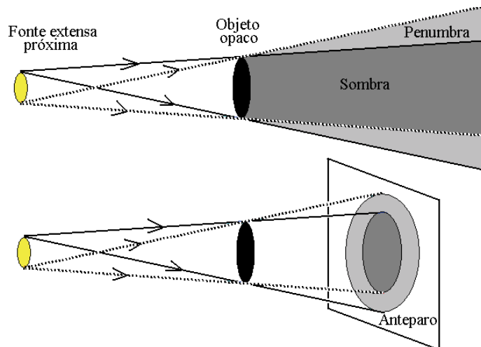
Fig. 6 - Sombra produzida por uma fonte extensa próxima e menor do que o objeto opaco que intercepta seus raios luminosos. A região de sombra é dominante sobre a região de penumbra, de forma que as bordas da sombra ficam mais nítidas. Essa nitidez é tanto maior quanto menor for a fonte.
