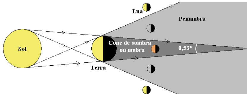
Fig. 13 - O diâmetro do cone de sombra da Terra perfaz cerca de 0,7 diâmetros terrestres ou 2,6 diâmetros lunares na região onde orbita a Lua.
