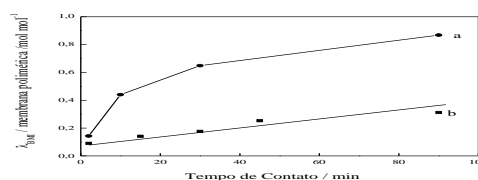
Figura 2. BMI / membrana polimérica razão molar em função do tempo de contato: (a) Nafion e (b) SPEEK.
