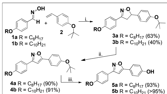
Esquema I. Rota sintética para obtenção dos fenóis 5 . i. NCS, Et 3 N, THF, HCl cat ; ii. MnO 2 , Tolueno; iii. HBr, AcOH, MeOH.
