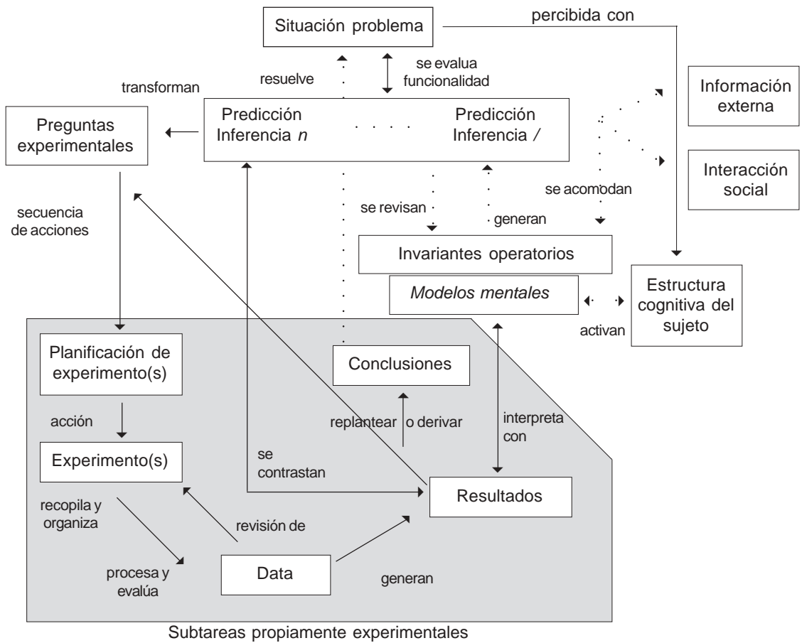
Figura 2 Modelo dinámico de Aprendizaje en los Trabajos de Laboratorio en Física (MATLaF)
