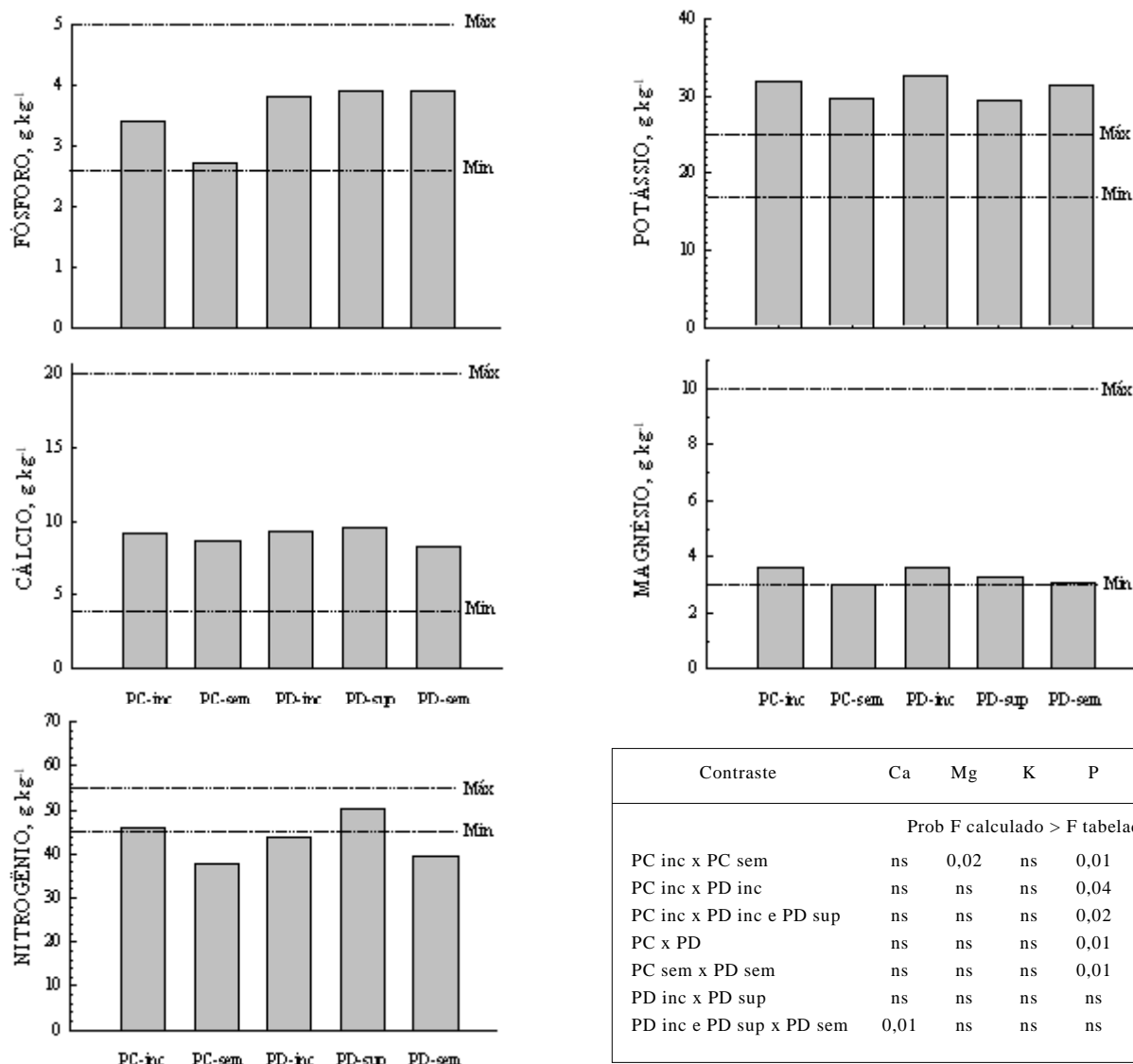
Figura 1. Teores de nutrientes no tecido da soja cultivada em plantio direto e preparo convencional em Latossolo Bruno Aluminico em Guarapuava - PR. PC inc = preparo convencional com calcário; PC sem = preparo convencional sem calcário; PD inc = plantio direto com calcário incorporado; PD sup = plantio direto com calcário superficial; PD sem = plantio direto sem calcário. Máx e Mín são os níveis máximos e mínimos adequados para cada elemento no tecido da soja.
